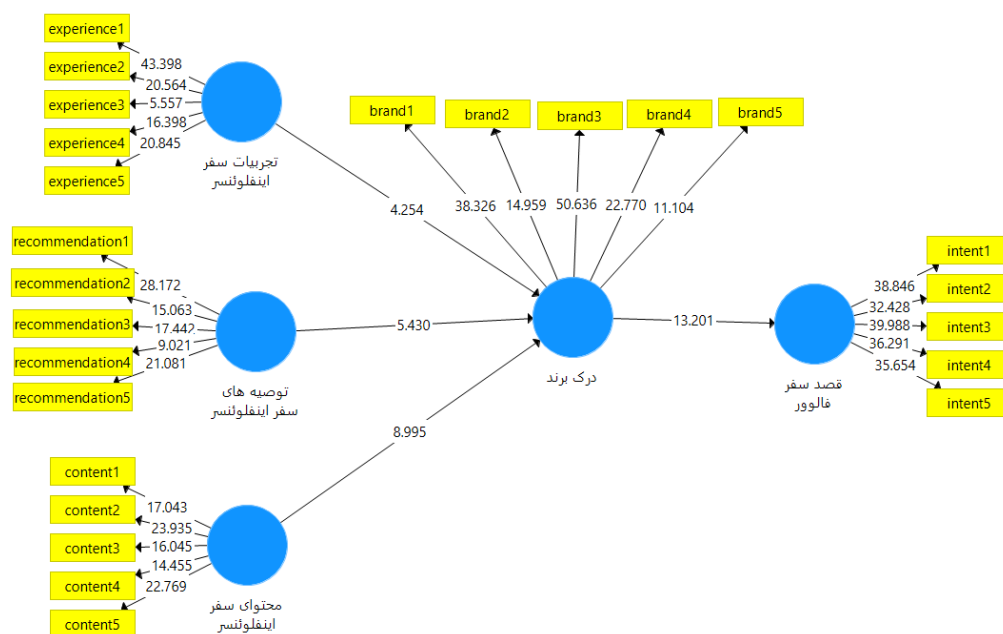
شکل ٢. مدل ساختاری نهایی پژوهش با مقادیر بارهای عاملی و ضرایب مسیر (بتا)
