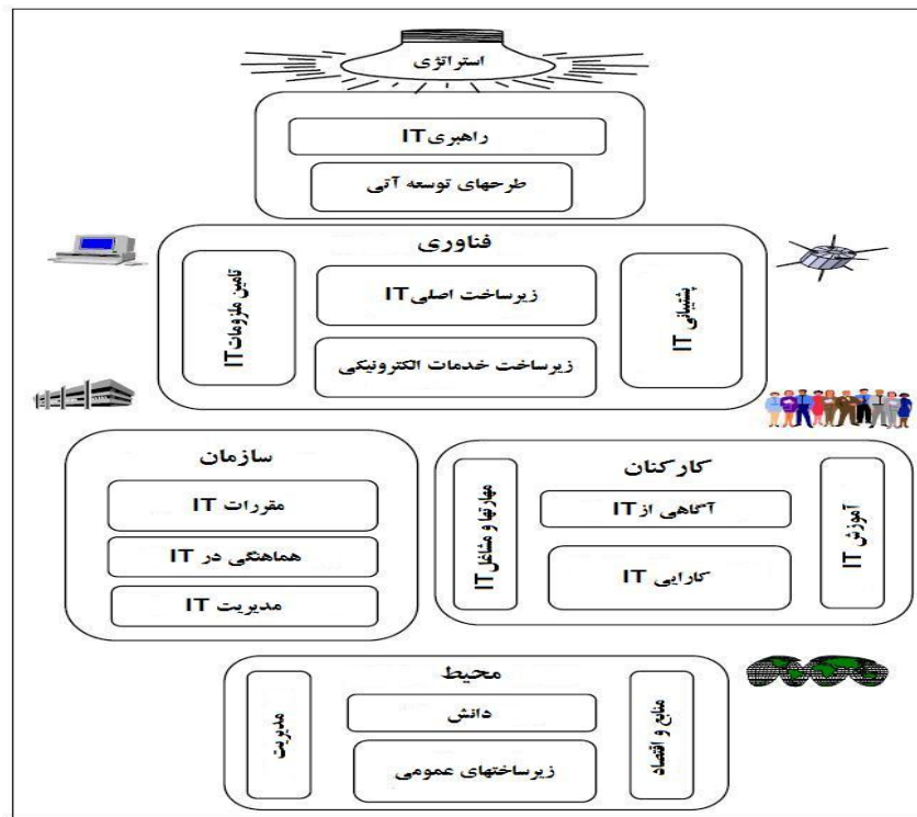
شکل ۲. مدل STOPE [۲۲]
